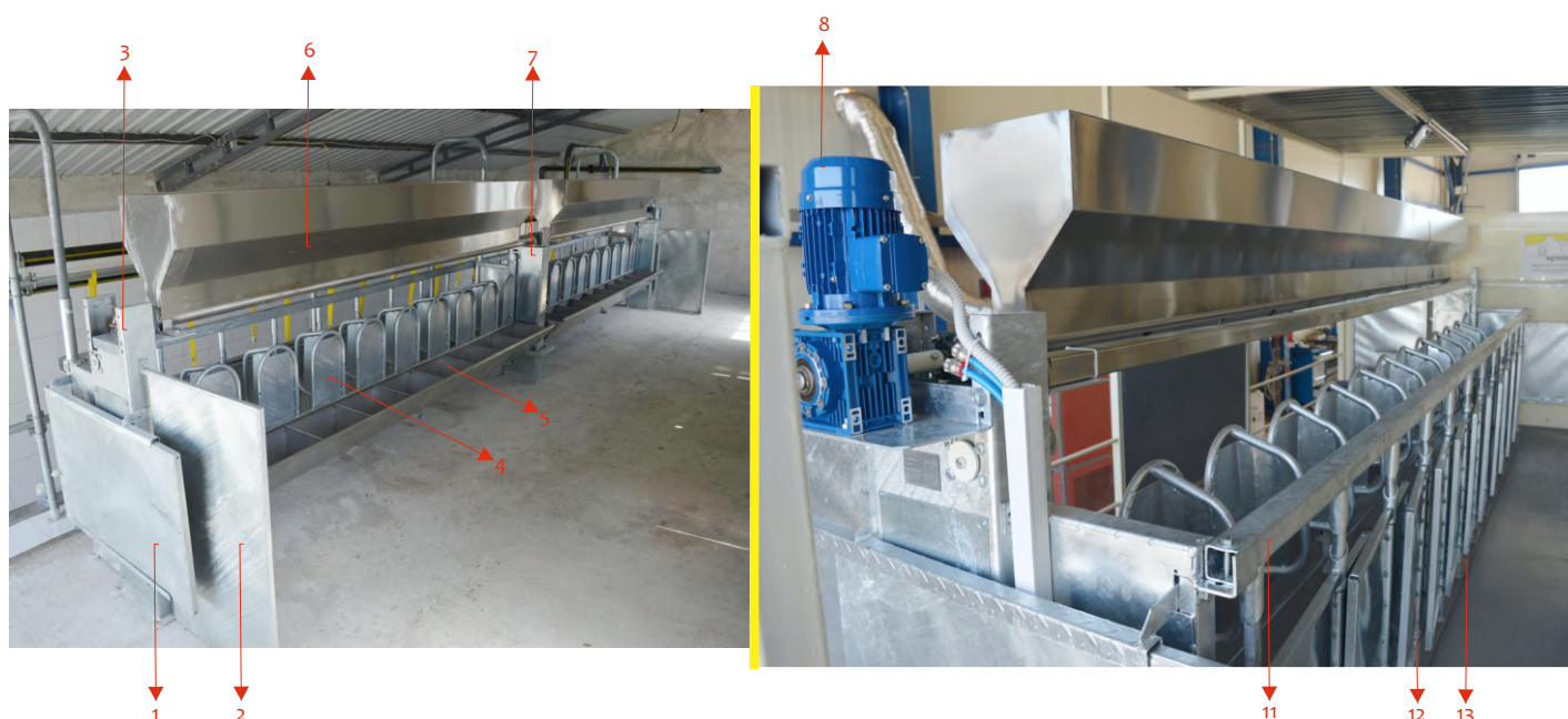
Partes del sistema neumático
