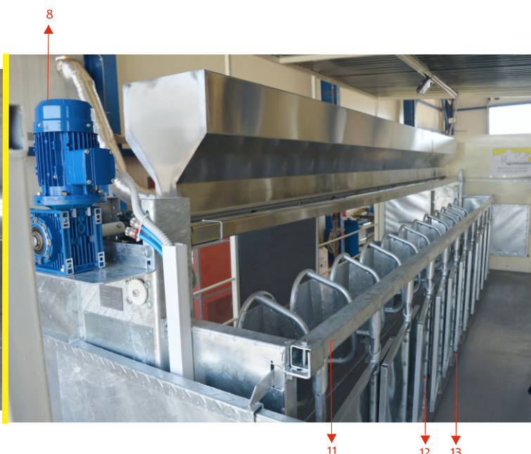
Μέρη αυτόματης τροφοδοσίας
